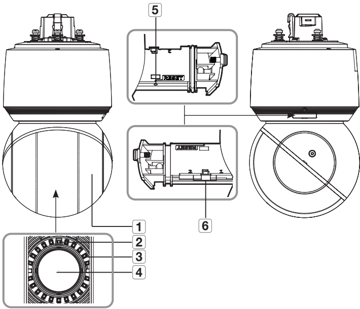
内部 (XNP-9250R/XNP-8250R/XNP-6400R)
