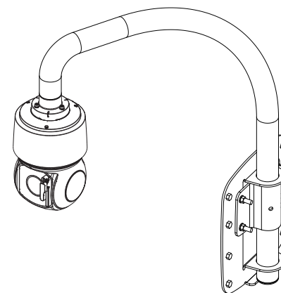
Montagem em parapeito (SBP-300LMW)
