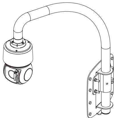
胸墙安装适配器 (SBP-300LMW)
