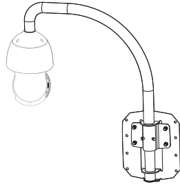
Parmaklık Montajı (SBP-300LM)
