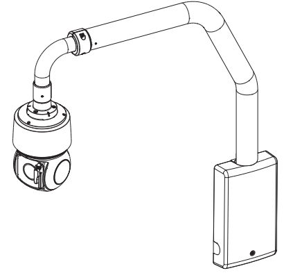
Parmaklık Montajı (SBP-156LMW)
