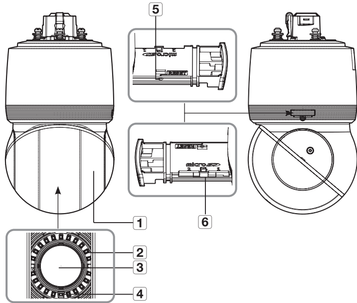
内部 (XNP-C9253R/XNP-C8253R/XNP-C6403R)
