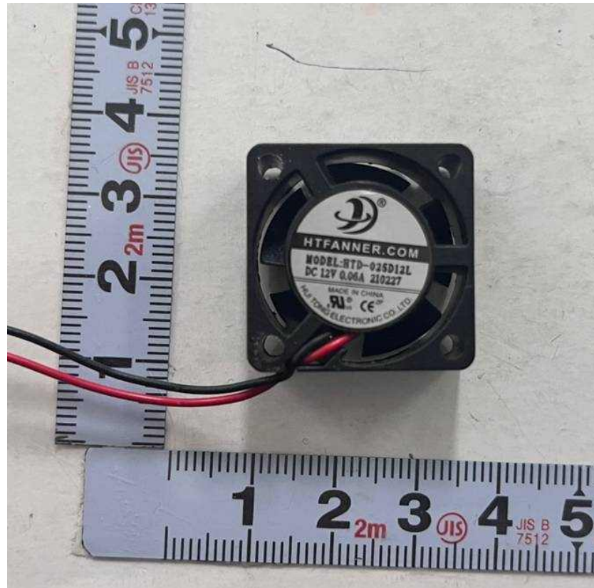
<Photo 10> DC Fan 2 bottom view
