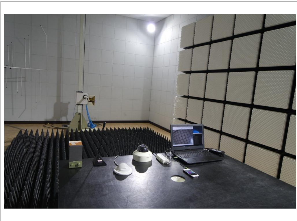
전 면 - PoE 모드
