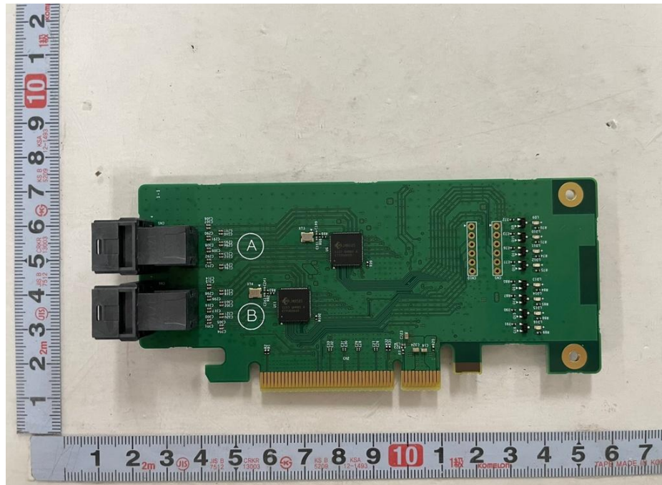
<사진 10> SW RAID CARD 전면
