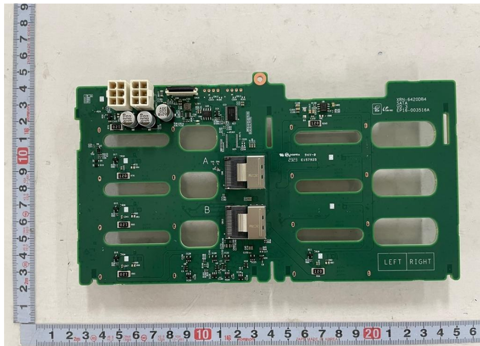
<사진 14> SATA-R 보드 전면
