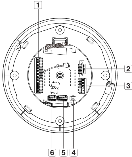
Vista interior de la base de instalación
