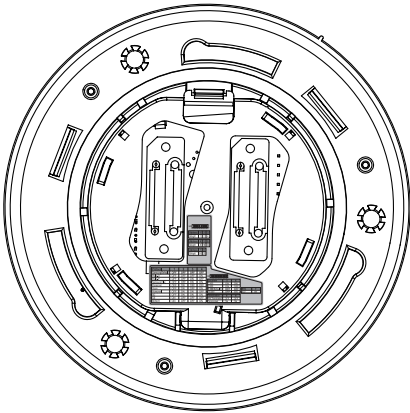
Vista inferior de la base de instalación
