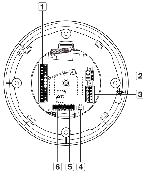
Innenansicht der Montagebasis
