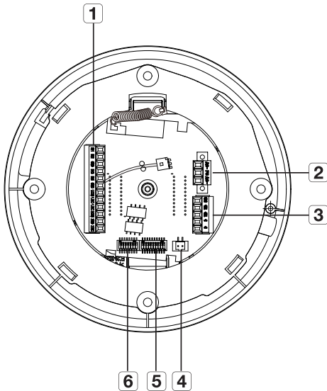
Vista interna della base di installazione
