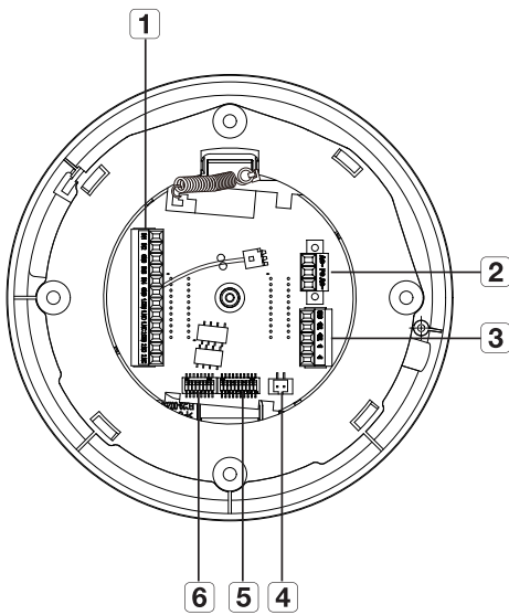
Izgled postolja za instalaciju sa unutrašnje strane.
