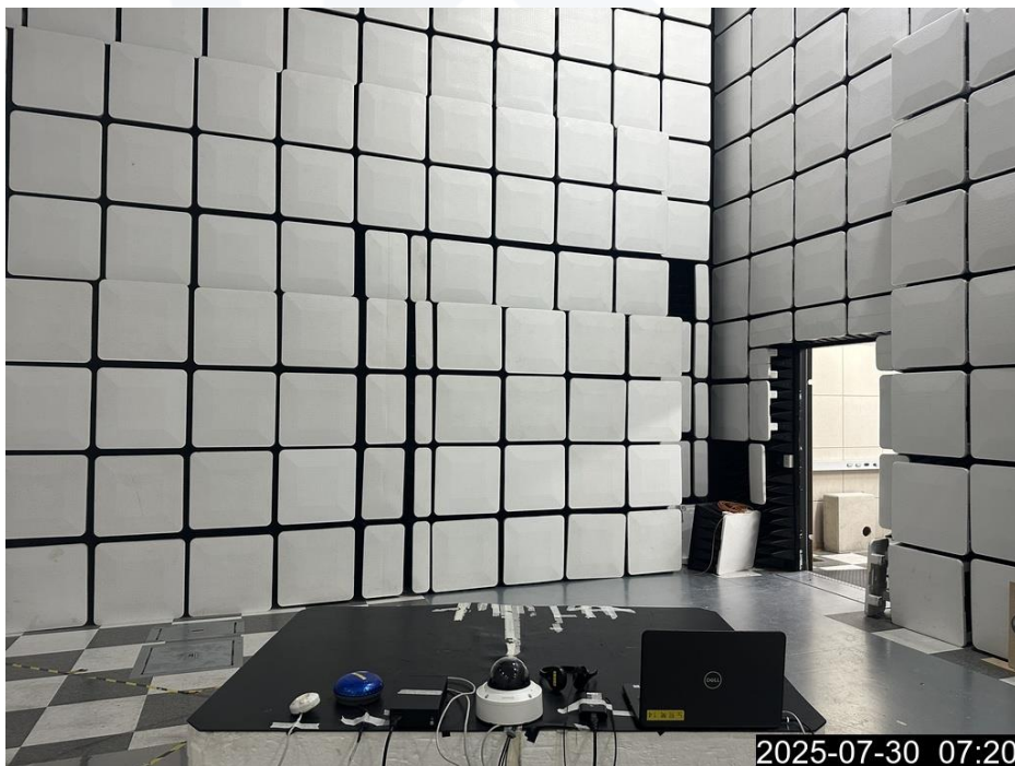
<방사성 방해-후면> Mode 2
