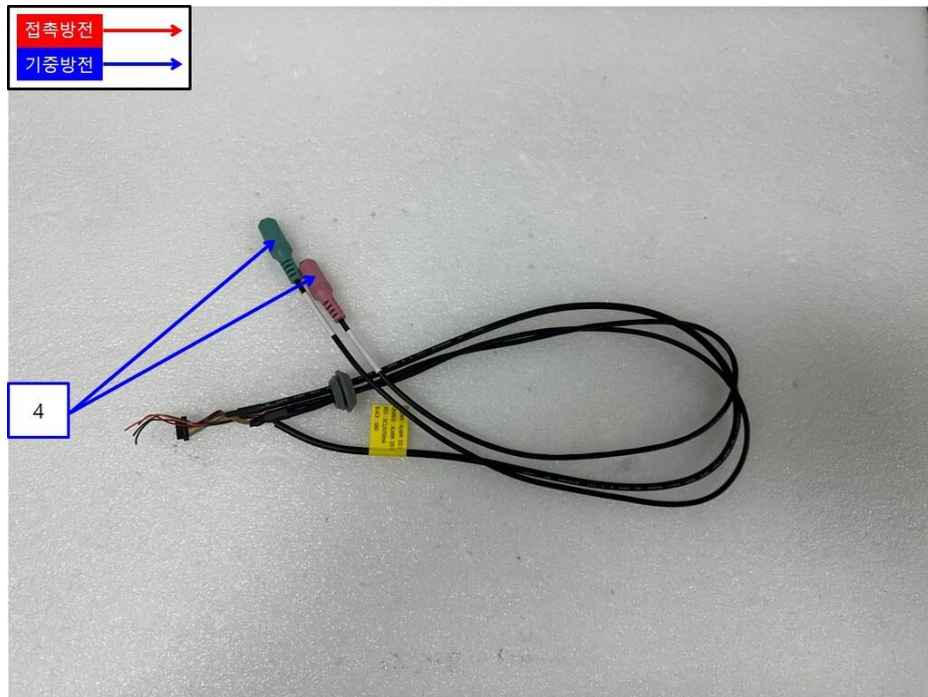
<정전기 인가부위-3> Mode 1, Mode 2
