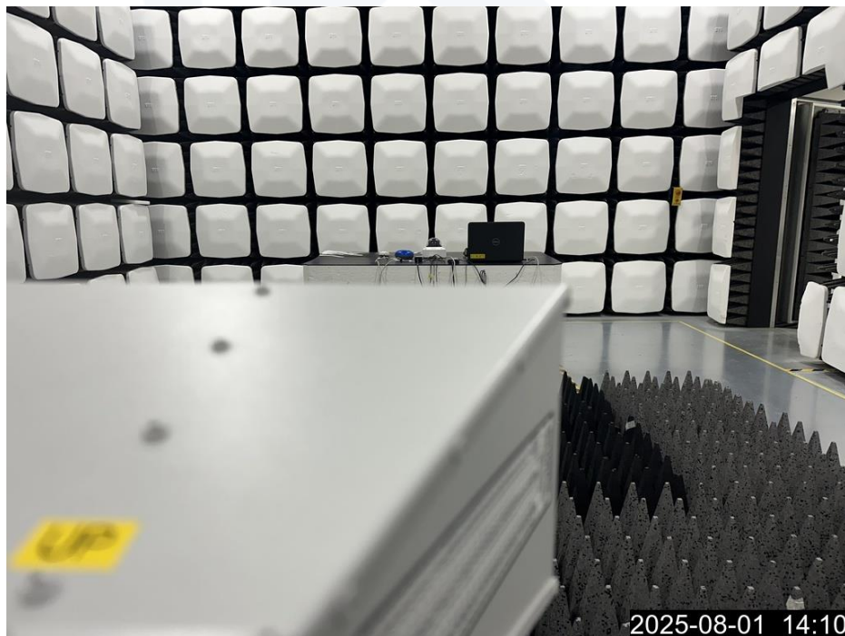
<방사성 방해(>1 GHz)-후면> Mode 1
