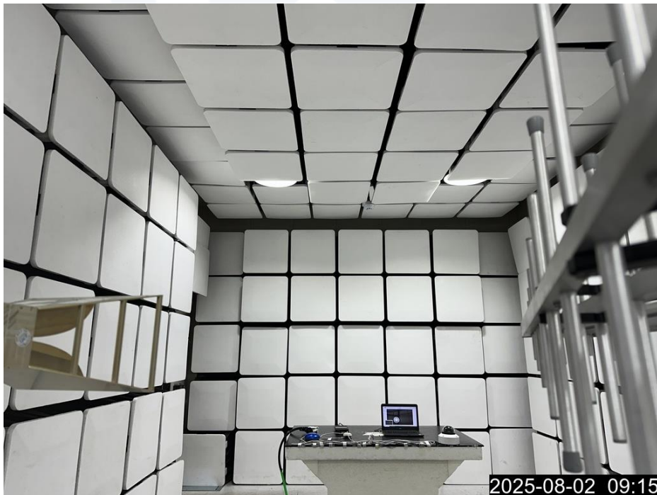
<방사성 RF 전자기장> Mode 2
