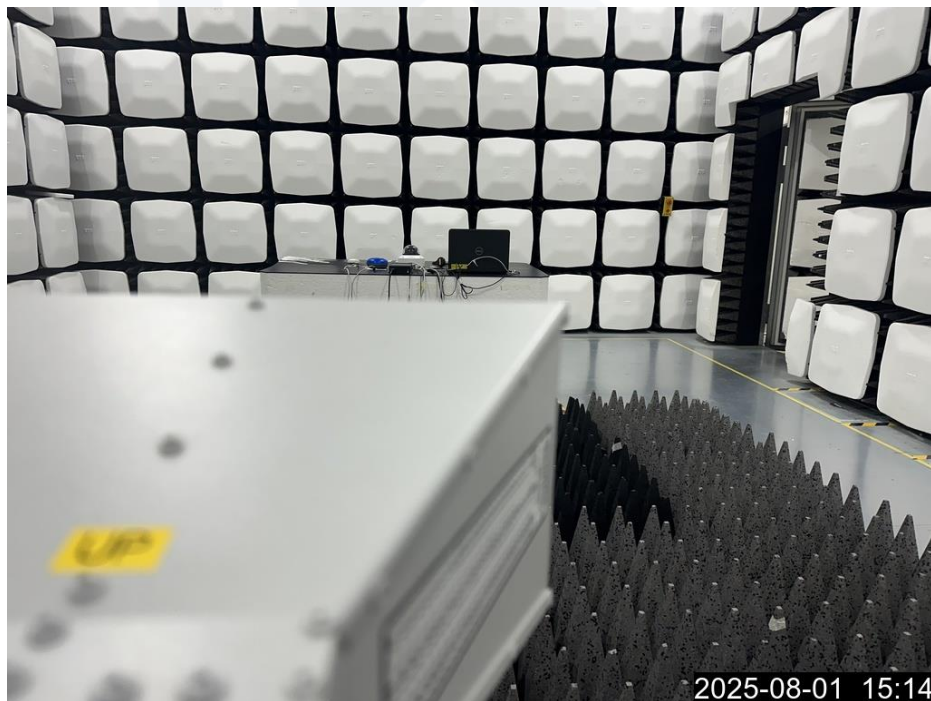
<방사성 방해(>1 GHz)-후면> Mode 2
