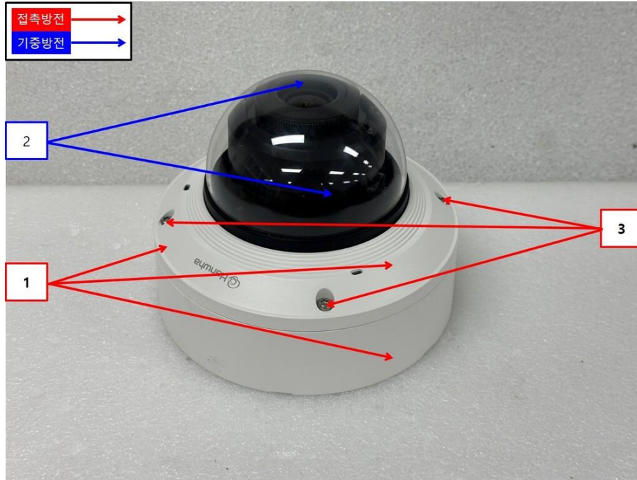
<정전기 인가부위-1> Mode 1, Mode 2
