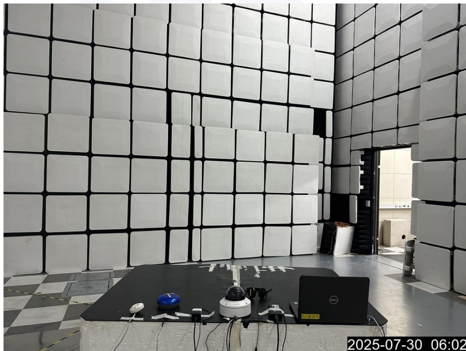
<방사성 방해-후면> Mode 1
