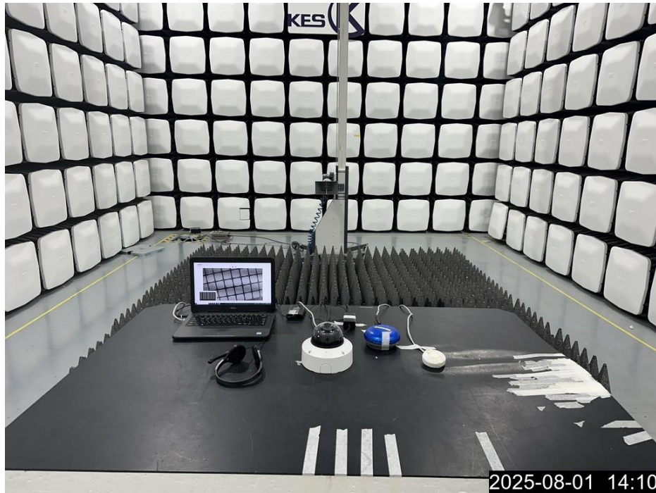
<방사성 방해(>1 GHz)-전면> Mode 1
