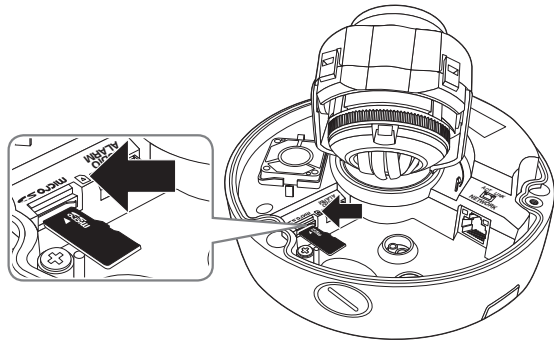
<PNV-9080R>
