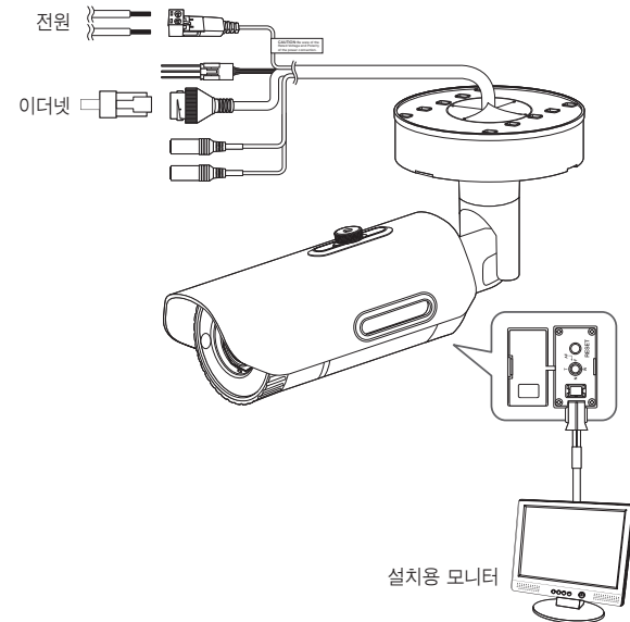
<PNO-9080R>
