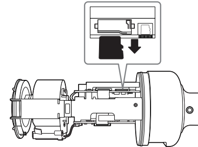
<PNO-9080R>
