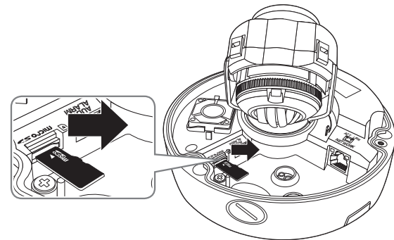
<PNV-9080R>
