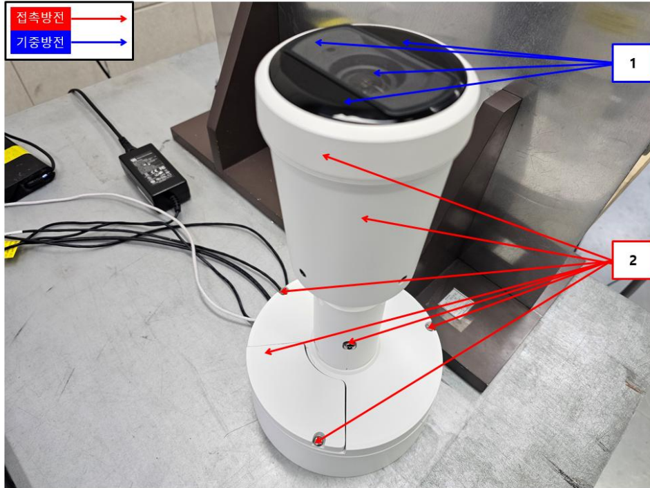
<정전기 인가부위-1>
