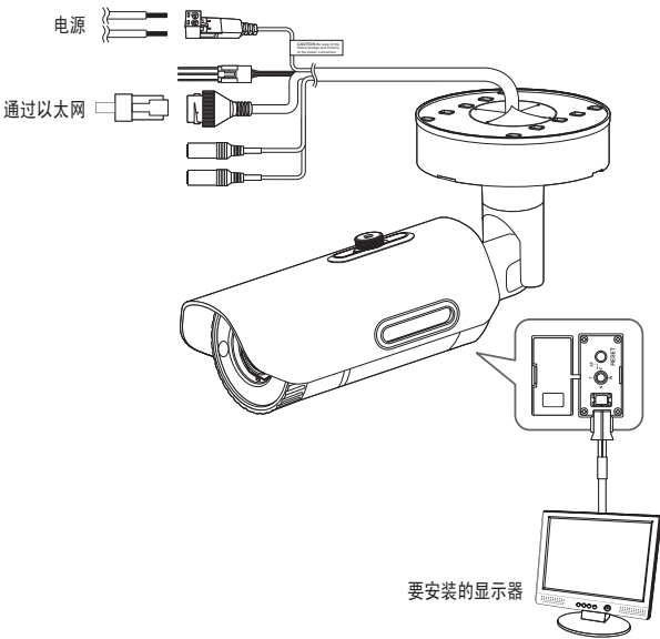
<PNO-9080R>
