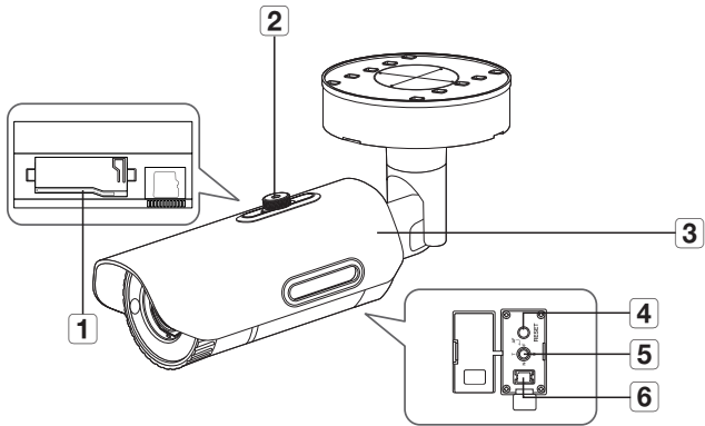
简图 (PNO-9080R)
