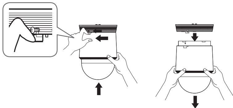
< 拆下摄像机 >
