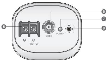
<DC12V (SCB-2005D)>
