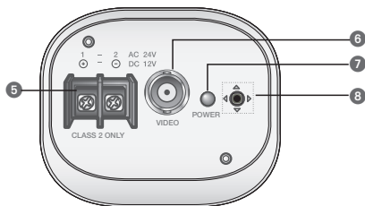
<AC24V/DC12V (SCB-2005)>
