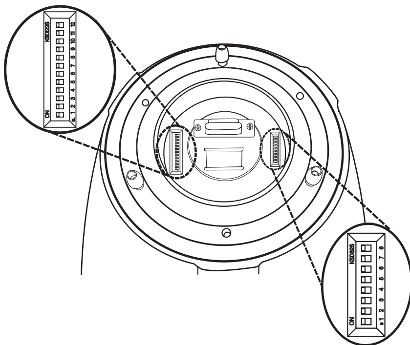
DIP-Schalter(SW1) für Kamera-ID
