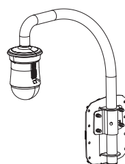
Brüstung-Montageset (SBP-300LM)
