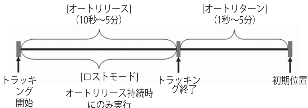
<オートトラッキングタイミング図>
