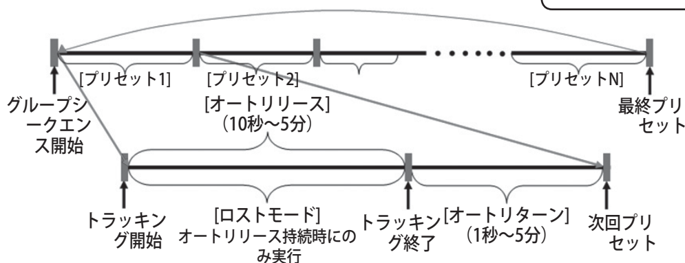
<グループシーケンスタイミング図>
