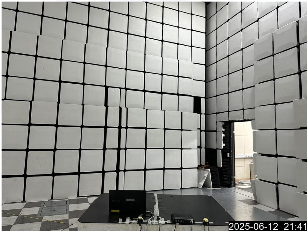
<방사성 방해-후면>
