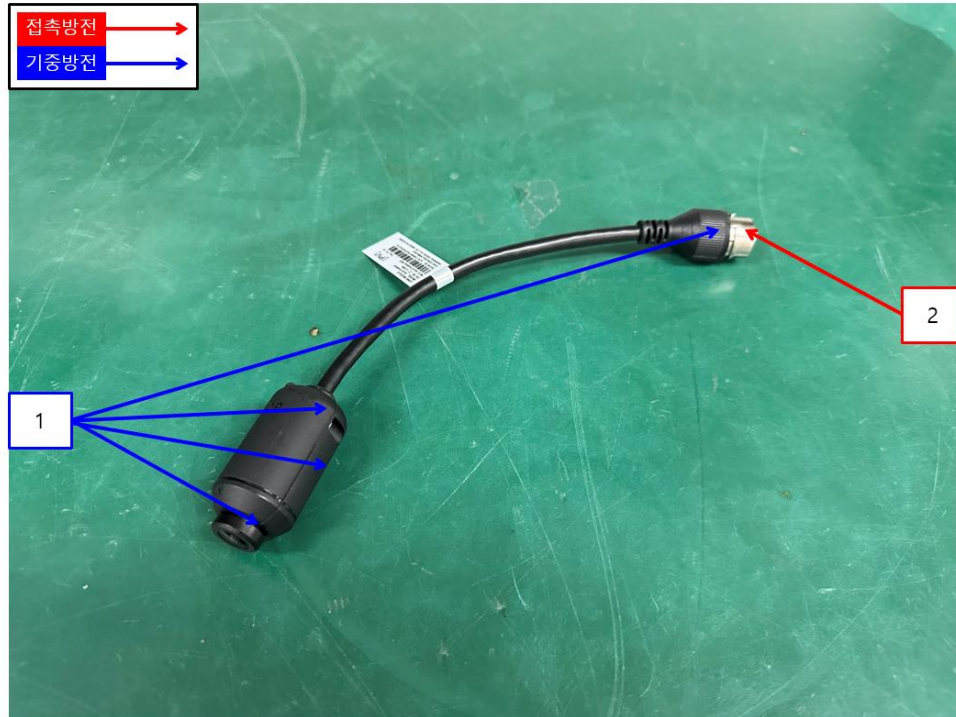
<정전기 인가부위-1>
