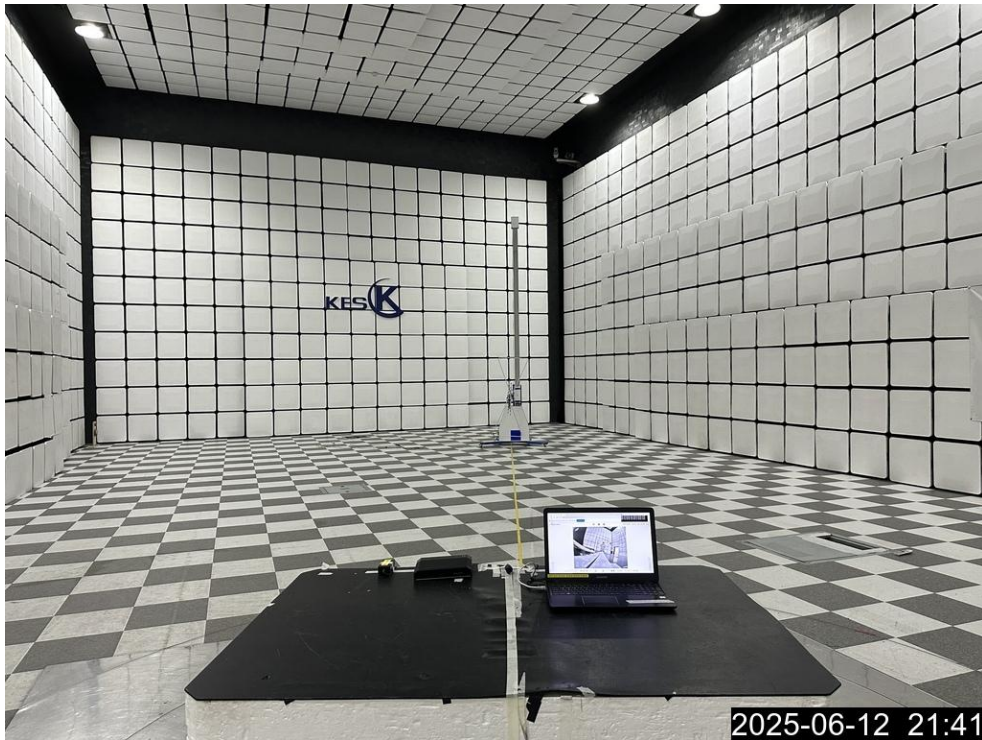
<방사성 방해-전면>
