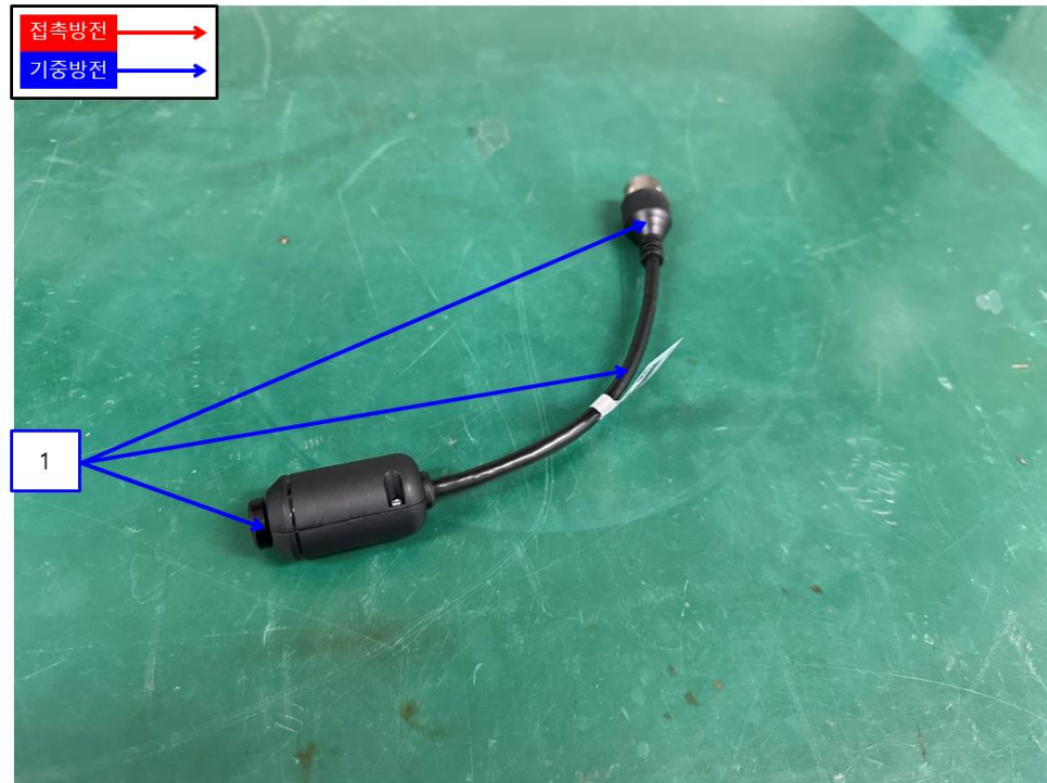
<정전기 인가부위-2>
