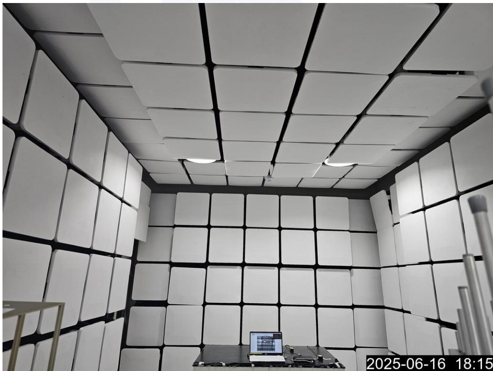
<방사성 RF 전자기장>
