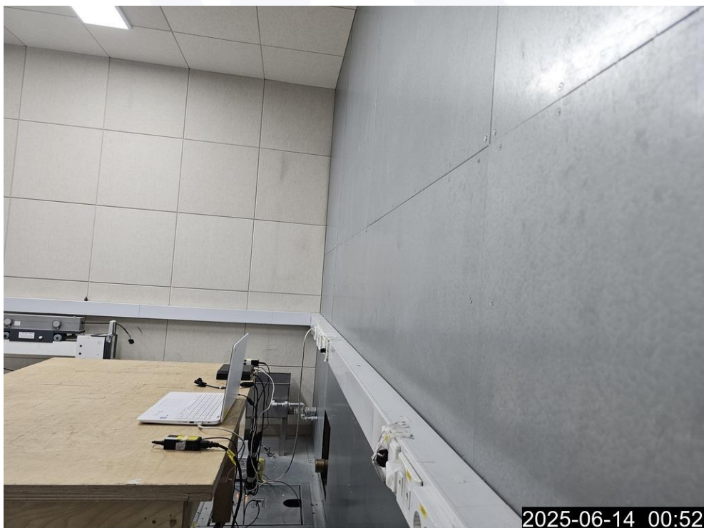
<전도성 방해-후면>
