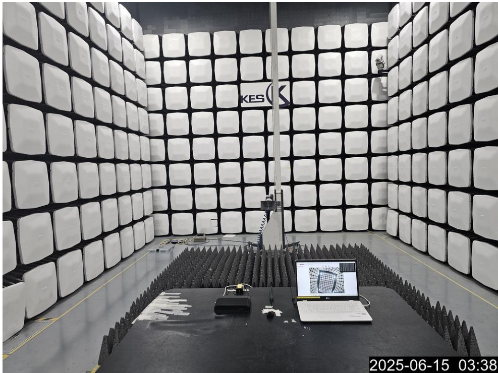
<방사성 방해(>1 GHz)-전면>
