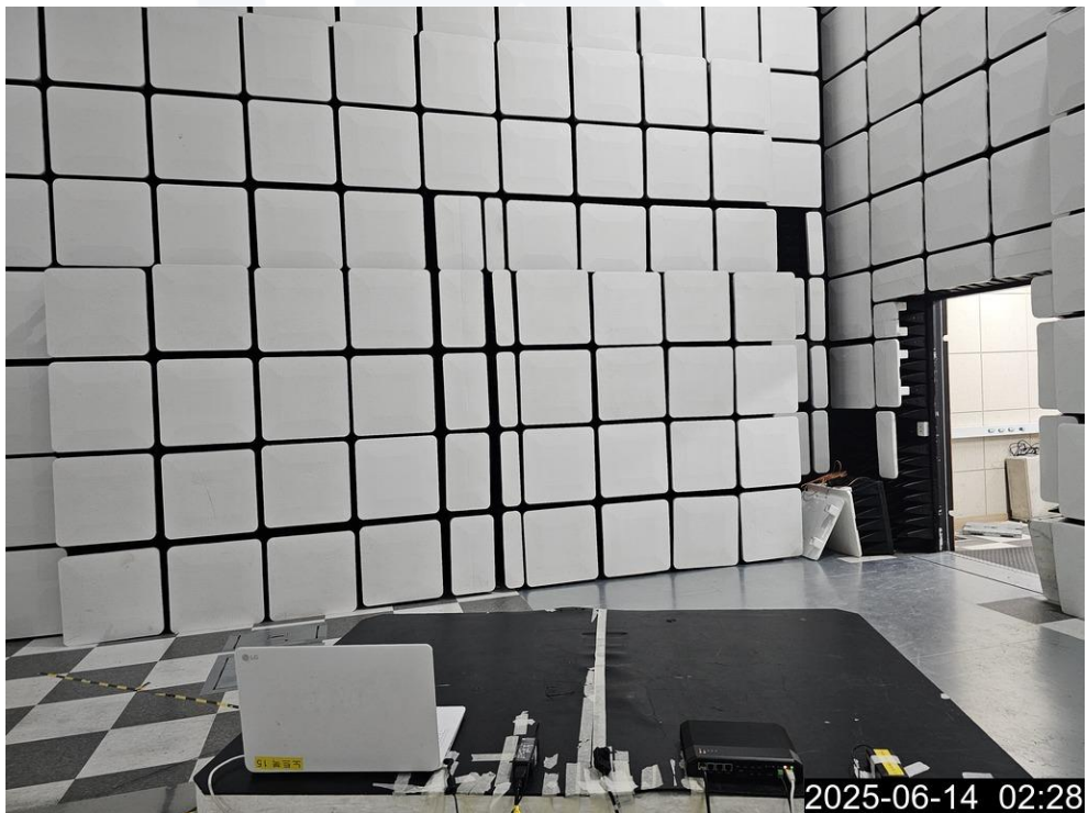
<방사성 방해-후면>
