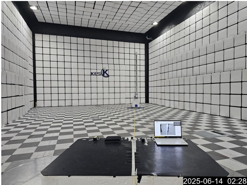
<방사성 방해-전면>
