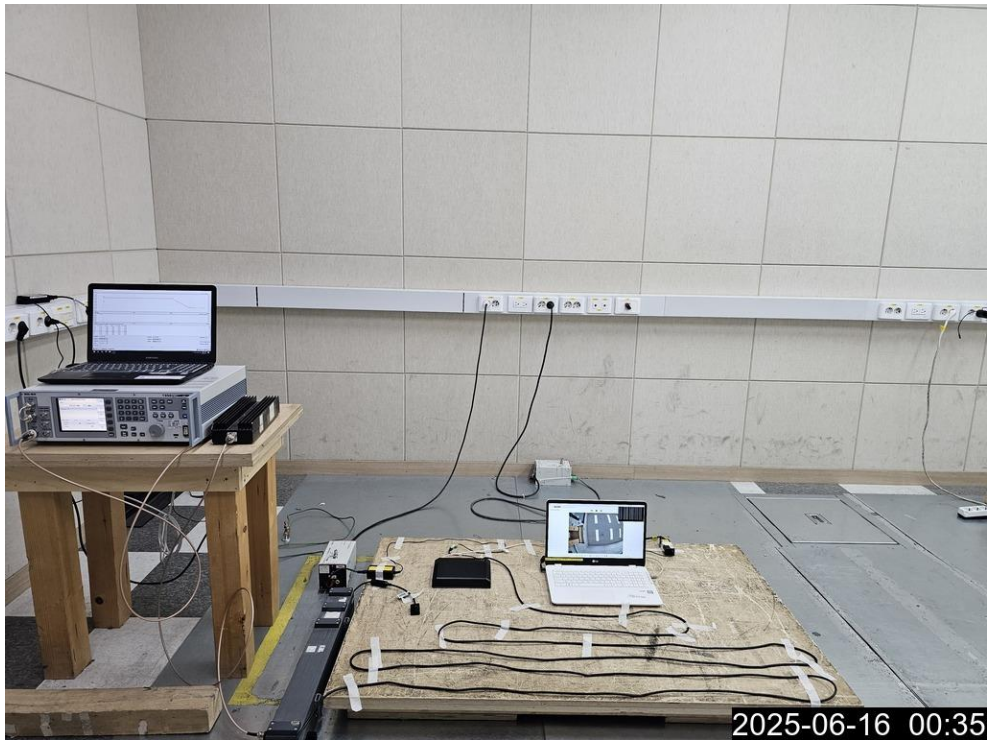
<전도성 RF 전자기장>
