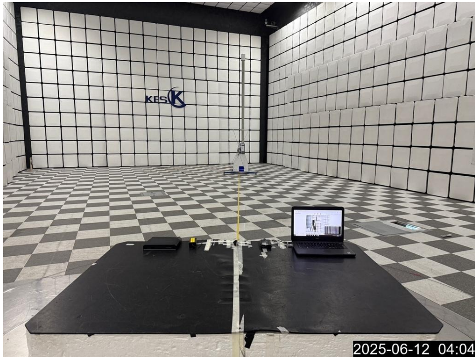
<방사성 방해-전면>
