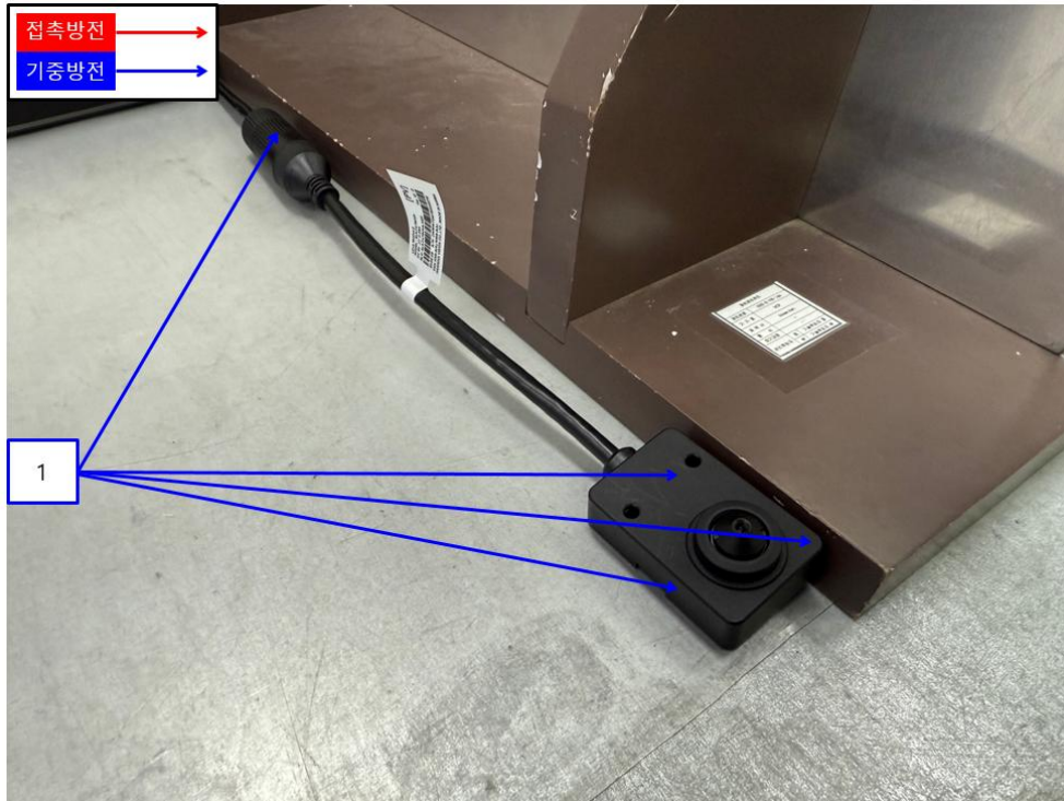
<정전기 인가부위-1>
