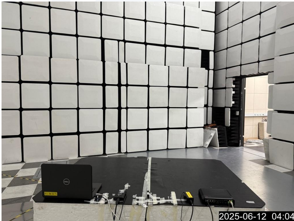
<방사성 방해-후면>
