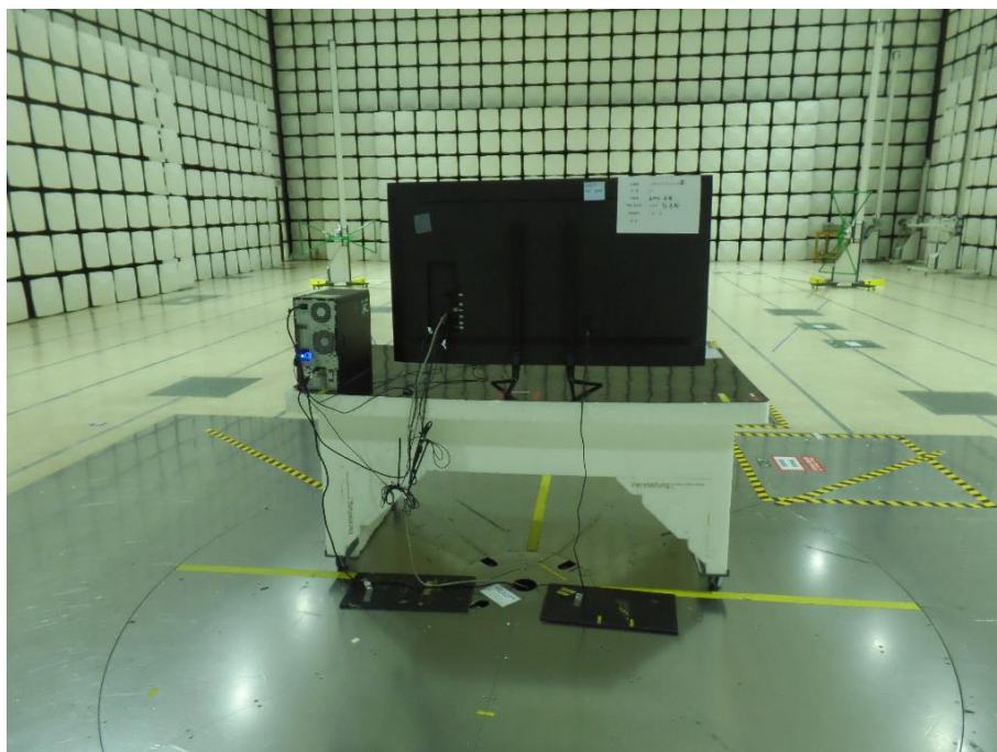
사진 4. 방사성 장애시험 [ 후면 ]
