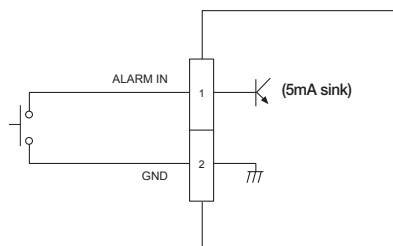
アラーム入力の配線図
