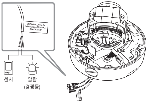
<SNV-8081R>
