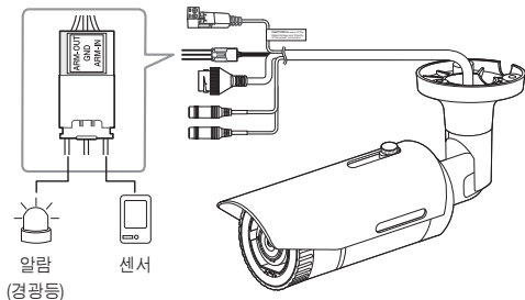
<SNO-8081R>
