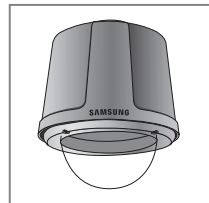
STH-360NPO Außenbereich- Leichtgehäuse (-20°~50°)
