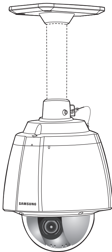
Montaż sufitowy (STB-300PP)
