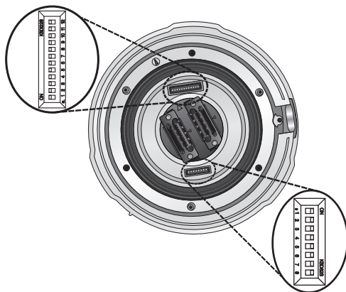
Chave DIP ID da câmera (SW1)
