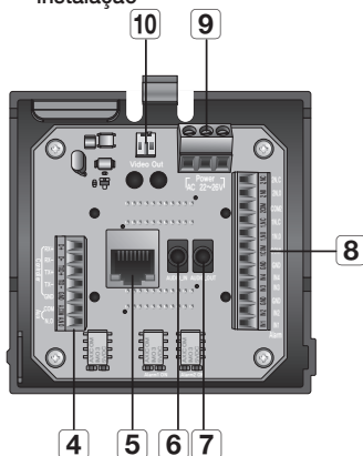
Visão interna da base de instalação
