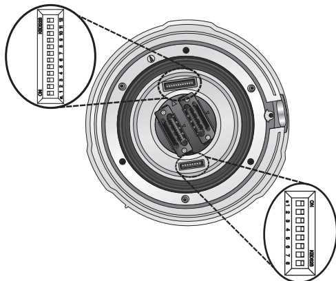
Conmutador DIP de ID de cámara (SW1)
