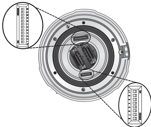
Commutateur DIP de l'ID de caméra (SW1)
