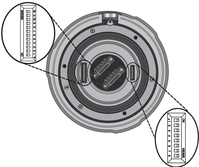
摄像机 ID DIP 开关 (SW1)
