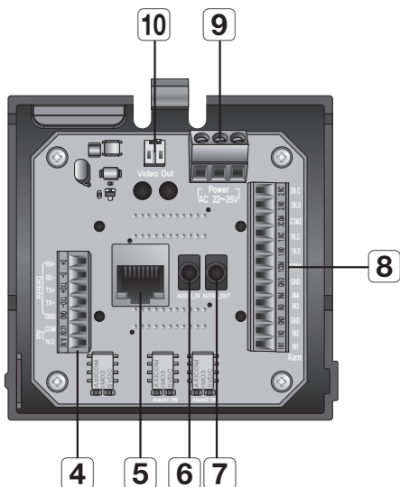
安装基座的内视图
