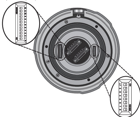
Spínač DIP pro ID kamery (SW1)
