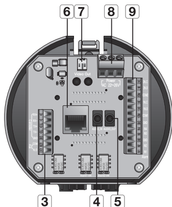
Vue interne de la base d'installation
