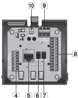
Vue interne de la base d'installation
