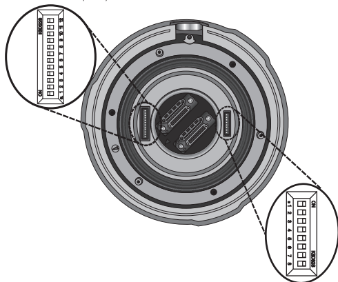
Commutateur DIP de l'ID de caméra (SW1)
