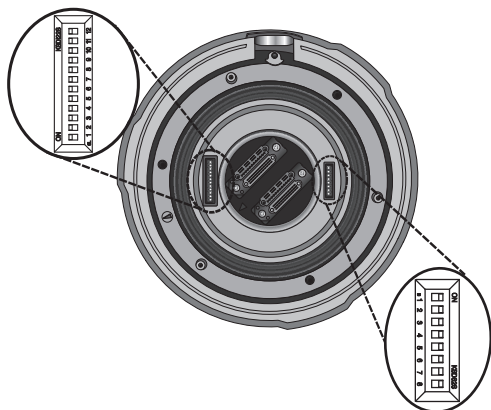
カメラIDのDIPスイッチ (SW1)
