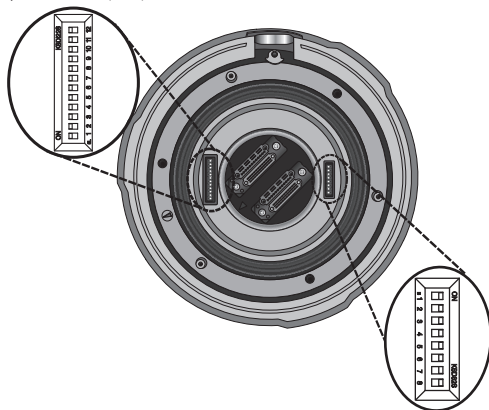
DIP переключатель ID камеры (SW1)
