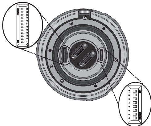
Conmutador DIP de ID de cámara (SW1)
