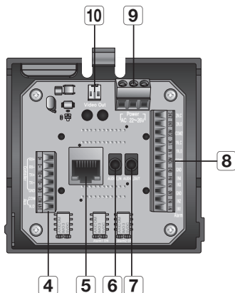
Vista interior de la base de instalación
