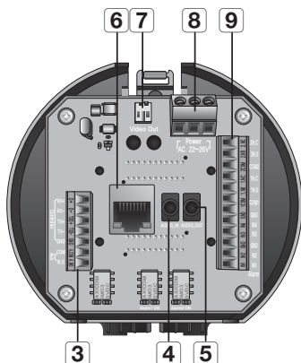
Vista interior de la base de instalación
