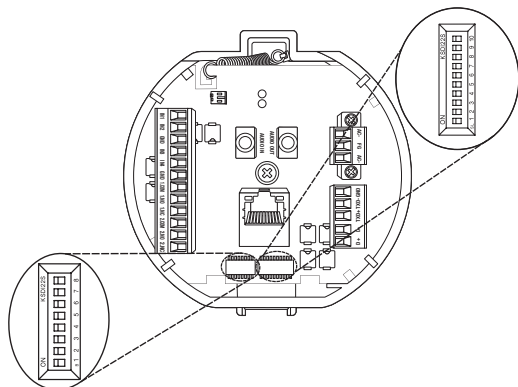
カメラIDのDIPスイッチ (SW1)
