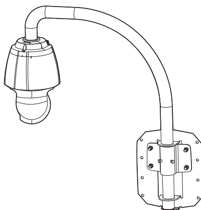
胸墙安装适配器 (SBP-300LM)
