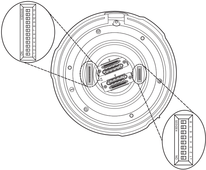
摄像机 ID DIP 开关 (SW1)
