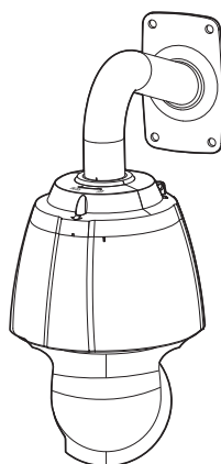
墙上安装适配器 (SBP-300WM)
