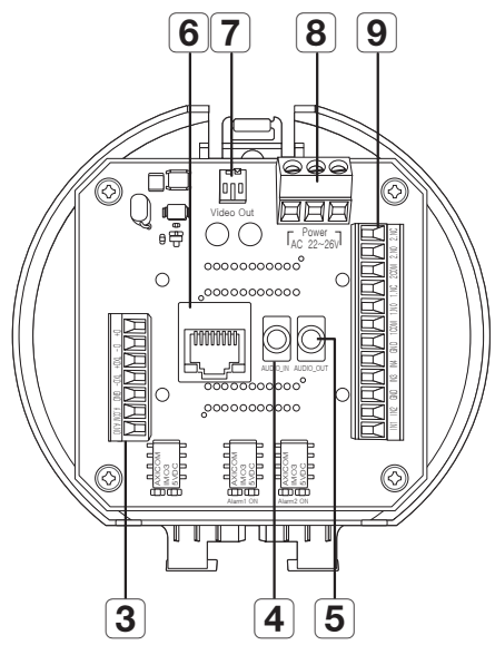
安装基座的内视图
