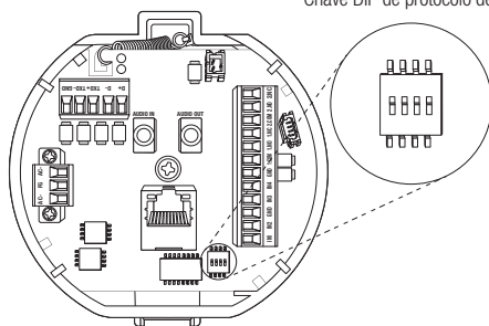
Chave DIP de protocolo de comunicação (SW1)
