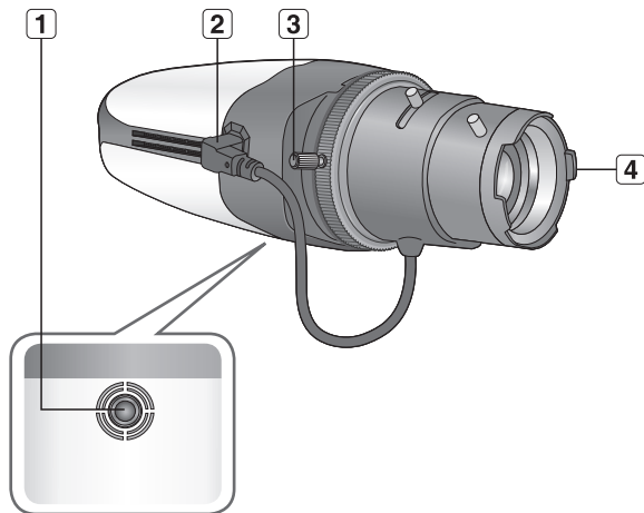
Pohled zvenčí
