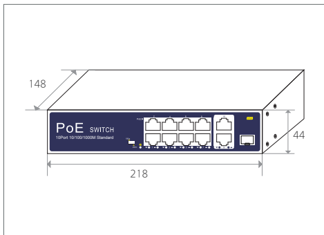
외관도
