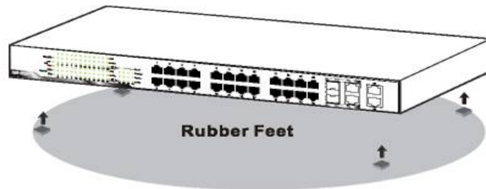
Figure 2.1 – 고무받침 부착
