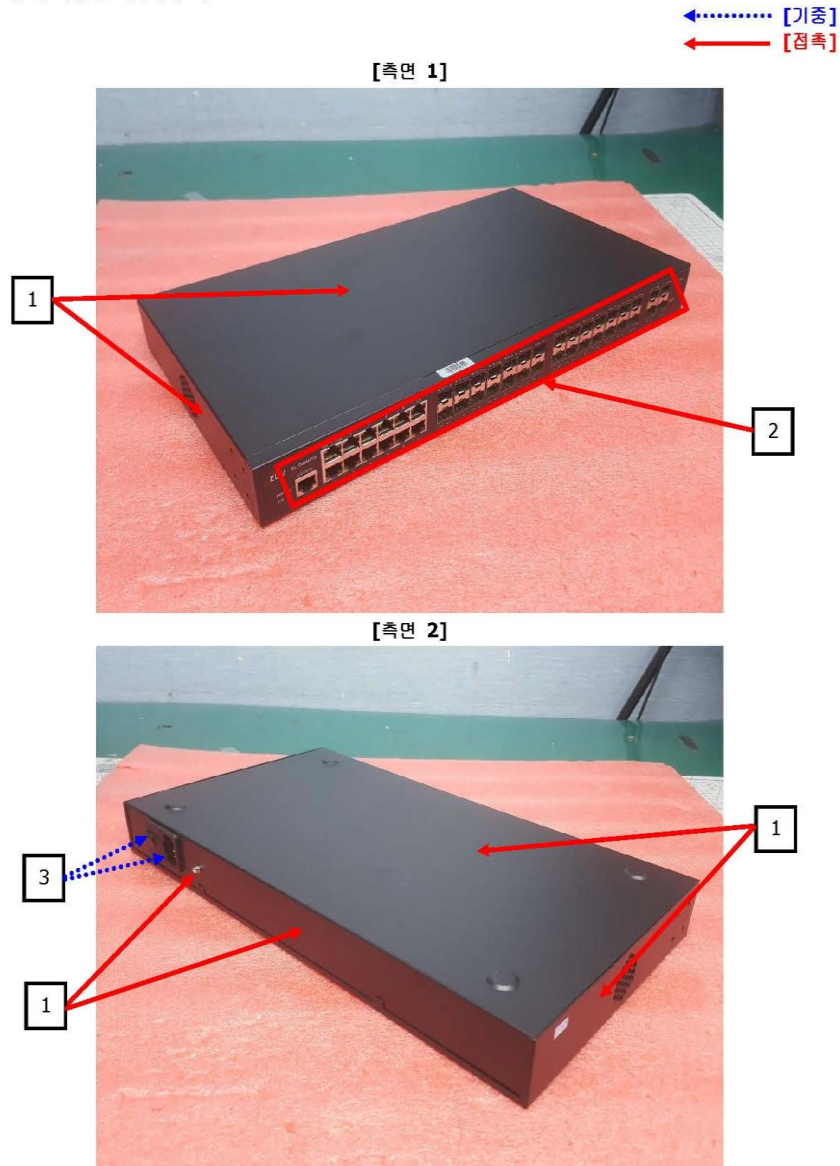
정전기방전 인가부위
