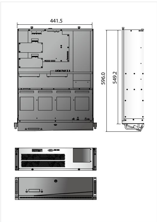
외관도 단위 : mm
