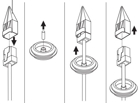
護蓋安裝器
