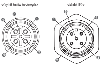
[Schemat styków złącza czytnika kodów kreskowych]
