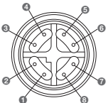
[Schemat styków złącza czytnika kodów kreskowych]
