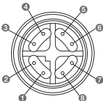
[Schemat styków złącza czytnika kodów kreskowych]
