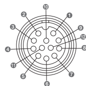
[Schemat styków złącza czytnika kodów kreskowych]
